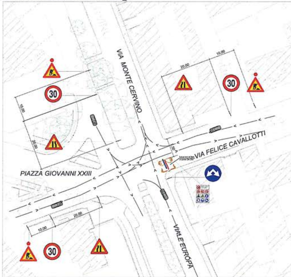
CANTIERIZZAZIONE TIPO - FASE 2a_3
