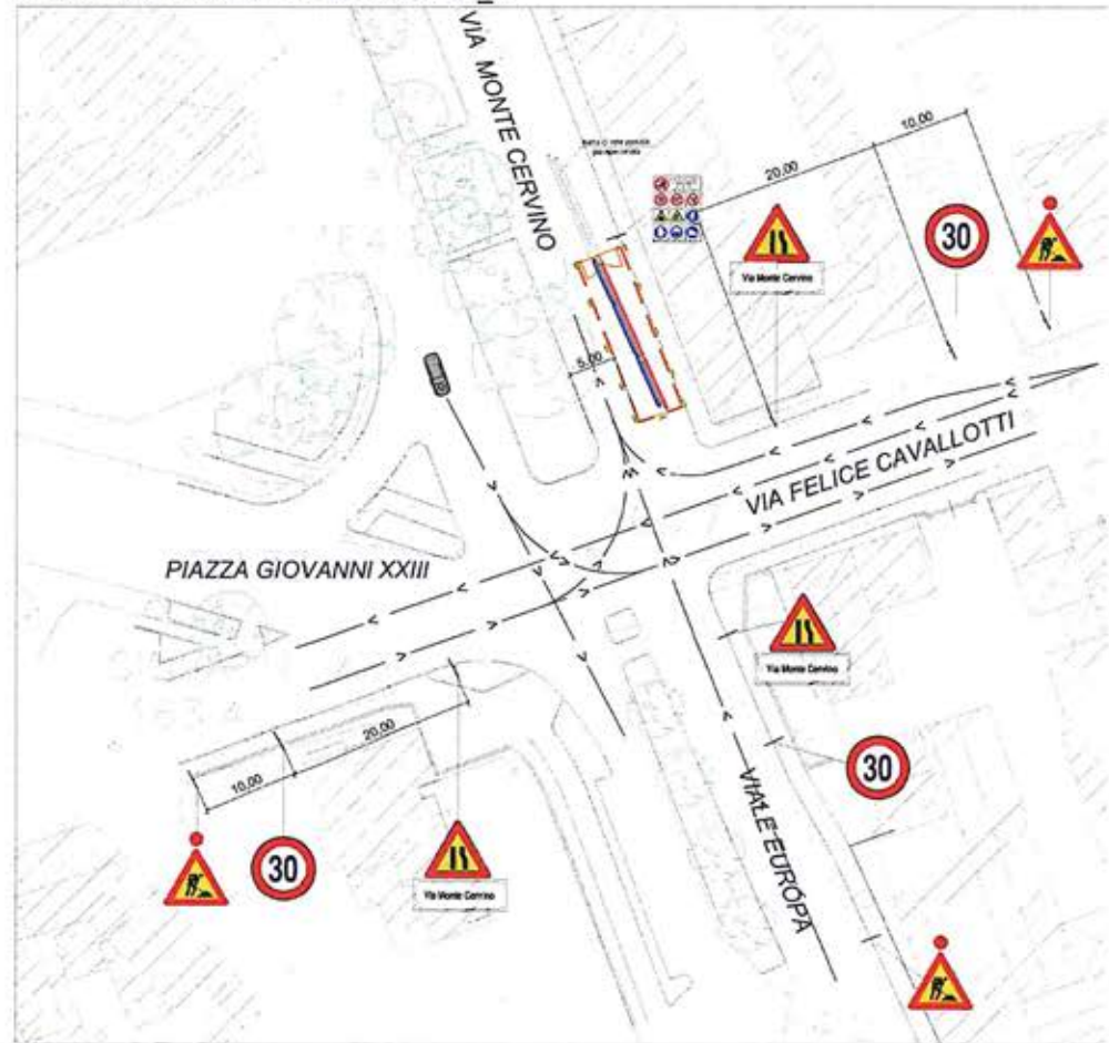
CANTIERIZZAZIONE TIPO - FASE 2a_4
