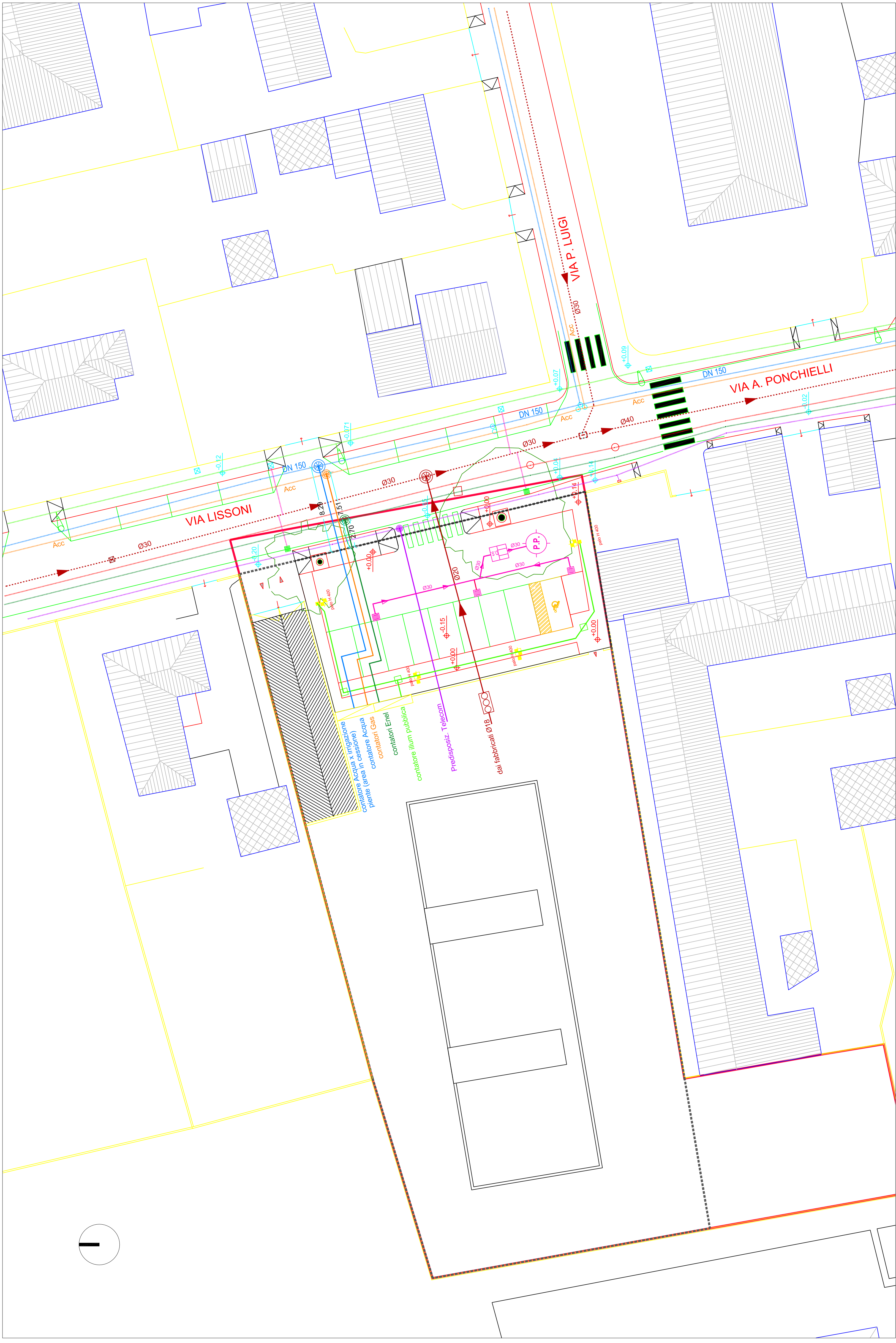
PLANIMETRIA 1:200
