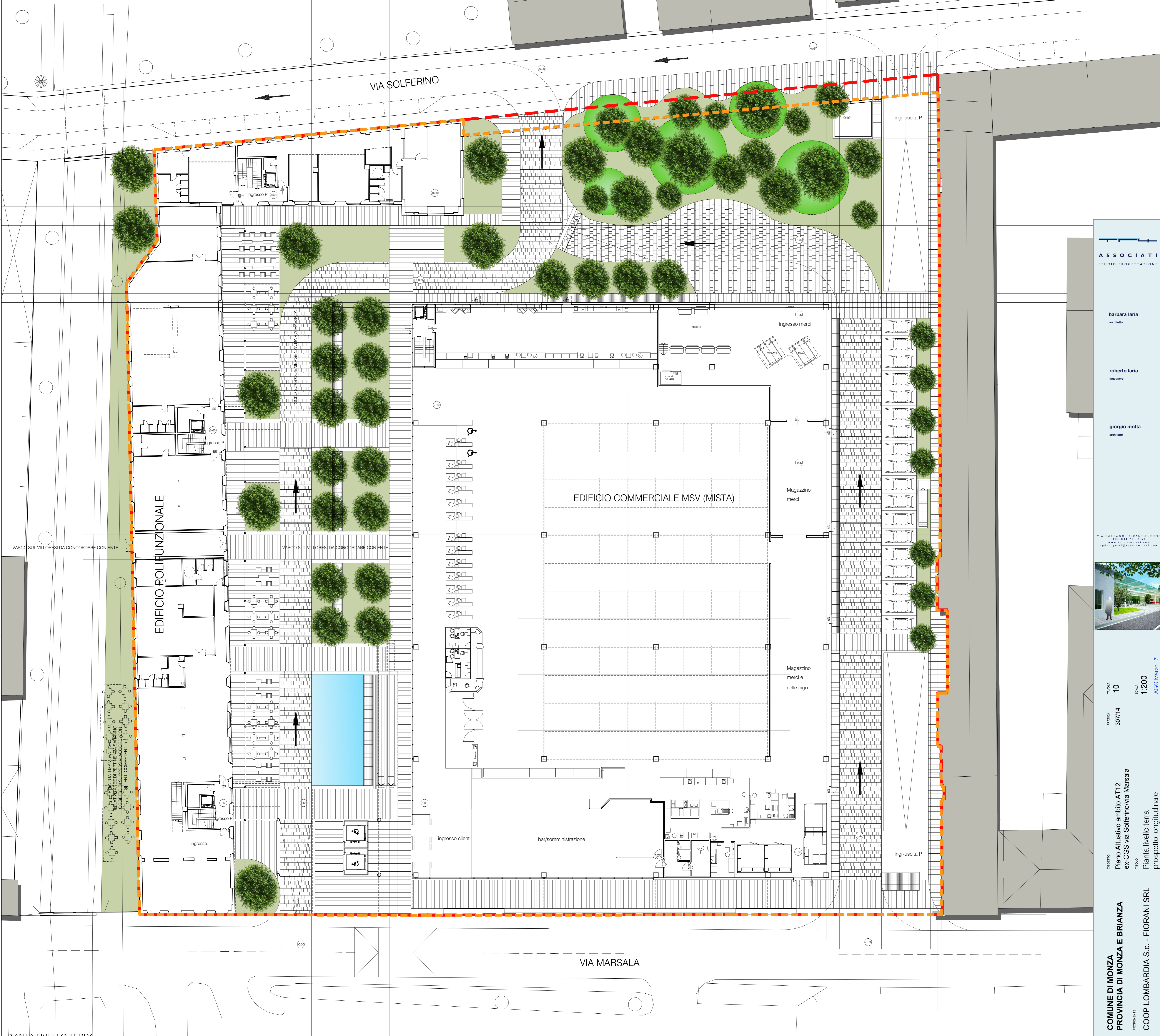
PIANTA LIVELLO TERRA
