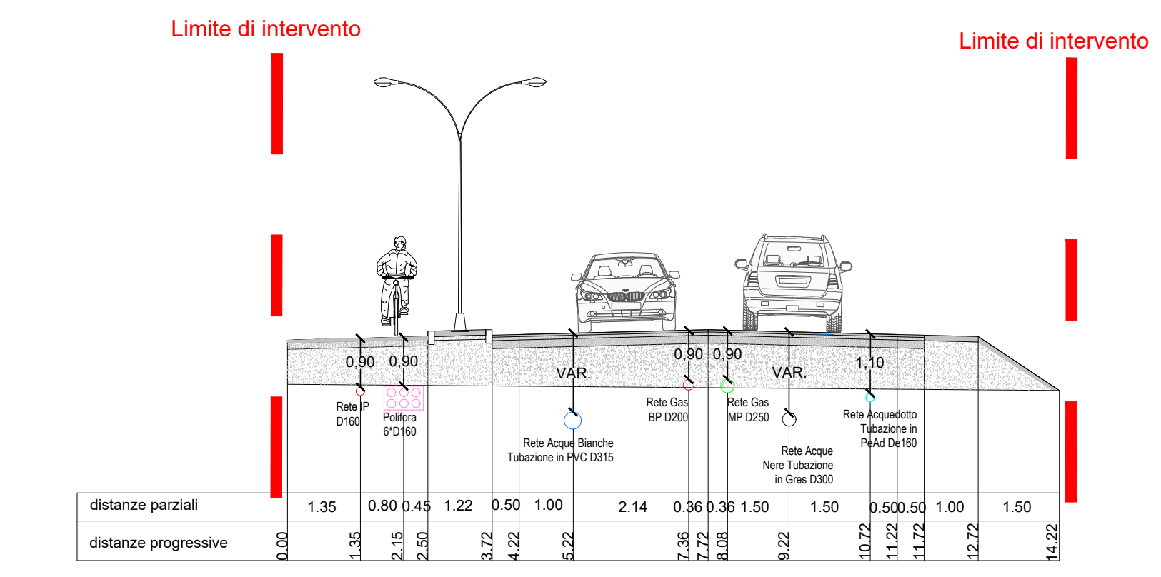
Sezione tipo A-A'
