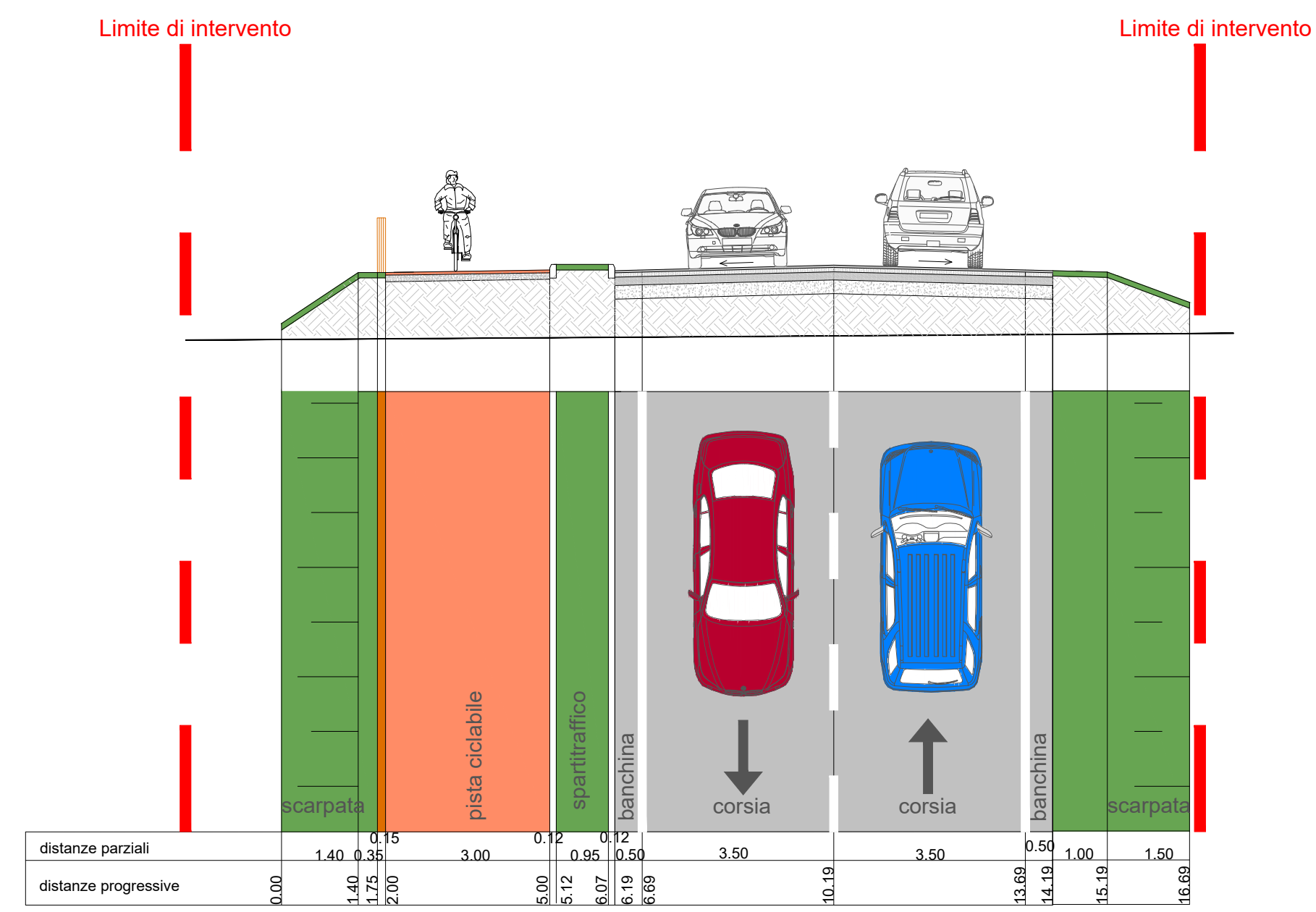
Sezione tipo A-A'
