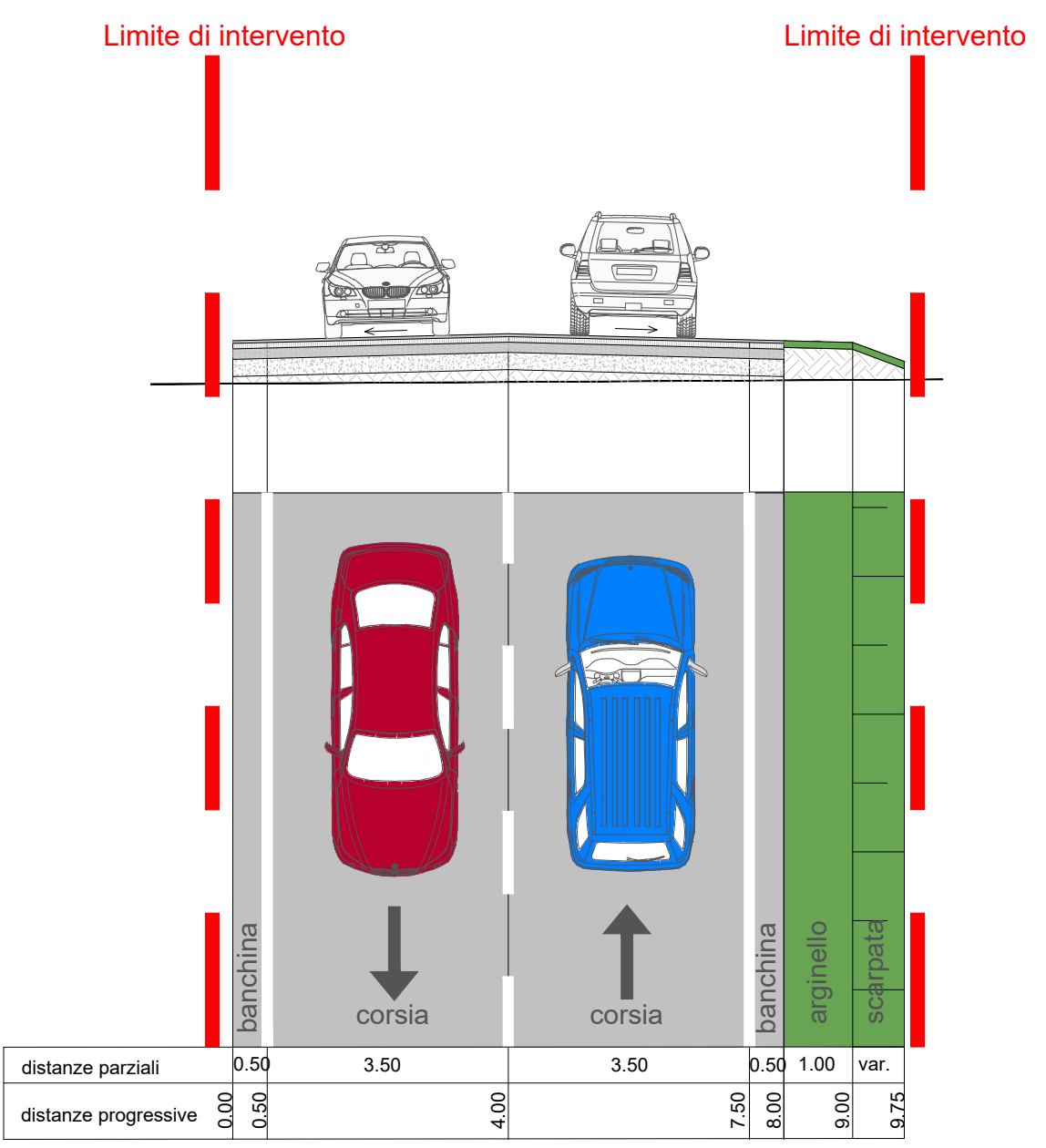
Sezione tipo B-B'
