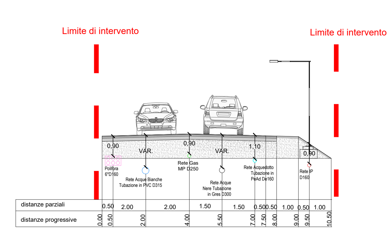
Sezione tipo B-B'
