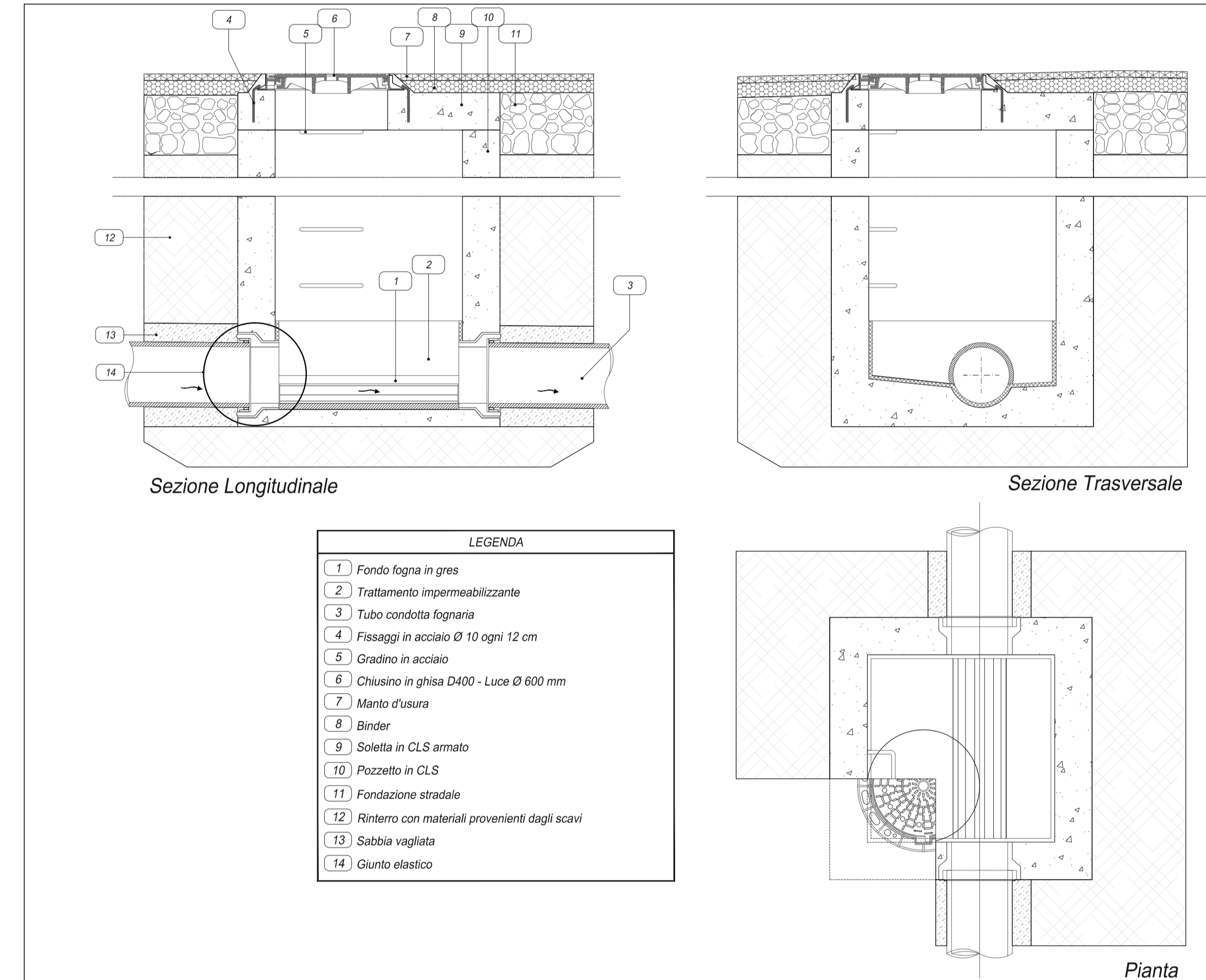
POZZETTO ISPEZIONE IN LINEA - DETTAGLI SCALA 1:20
